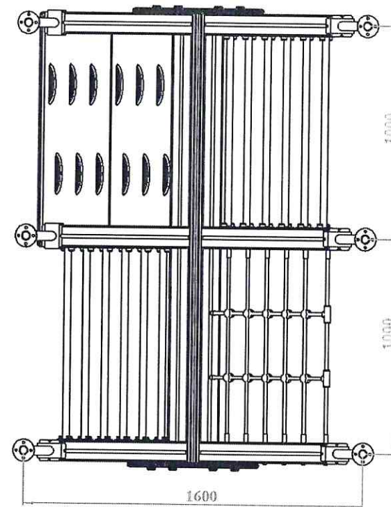
21.Схема бетонирования.
